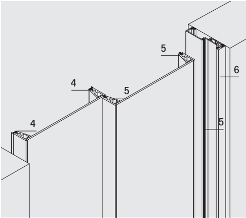
composizione con pannelli fuori luce senza montanti laterali composition out of the opening without side runners
