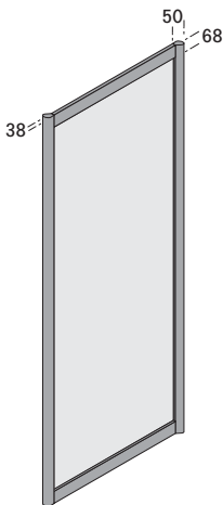
specchiatura intera / full height glass pag 94
