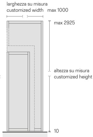
Dimensioni pannelli a libro e battenti Folding and swing panel dimensions
