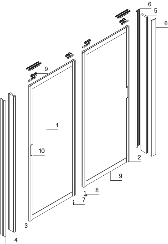
specchiatura intera / full height glass pag 94
